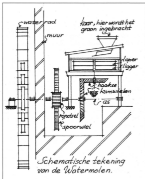
Afbeelding 3. Schematische tekening van de watermolen.
